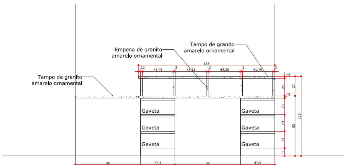
VISTA POSTERIOR ESCALA 1:25
