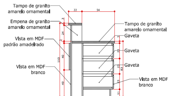
CORTE BB ESCALA 1:25
