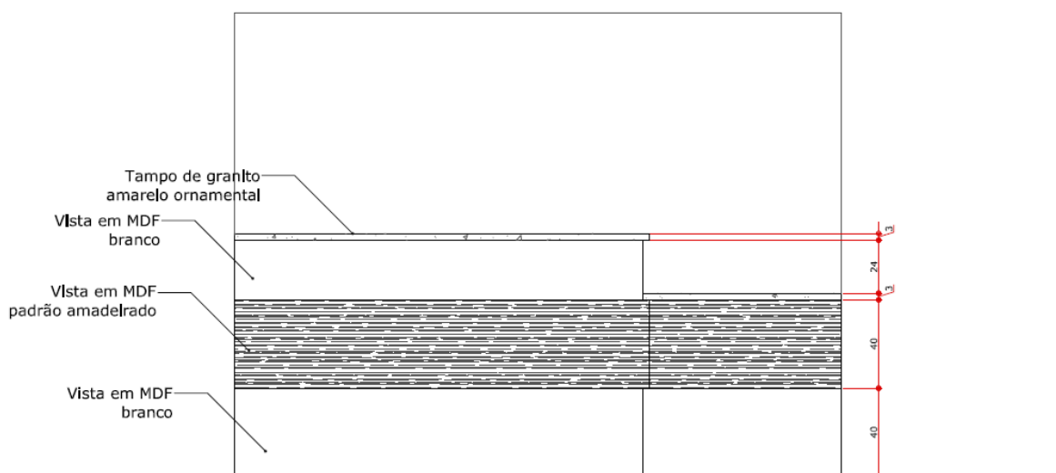
VISTA FRONTAL ESCALA 1:25
