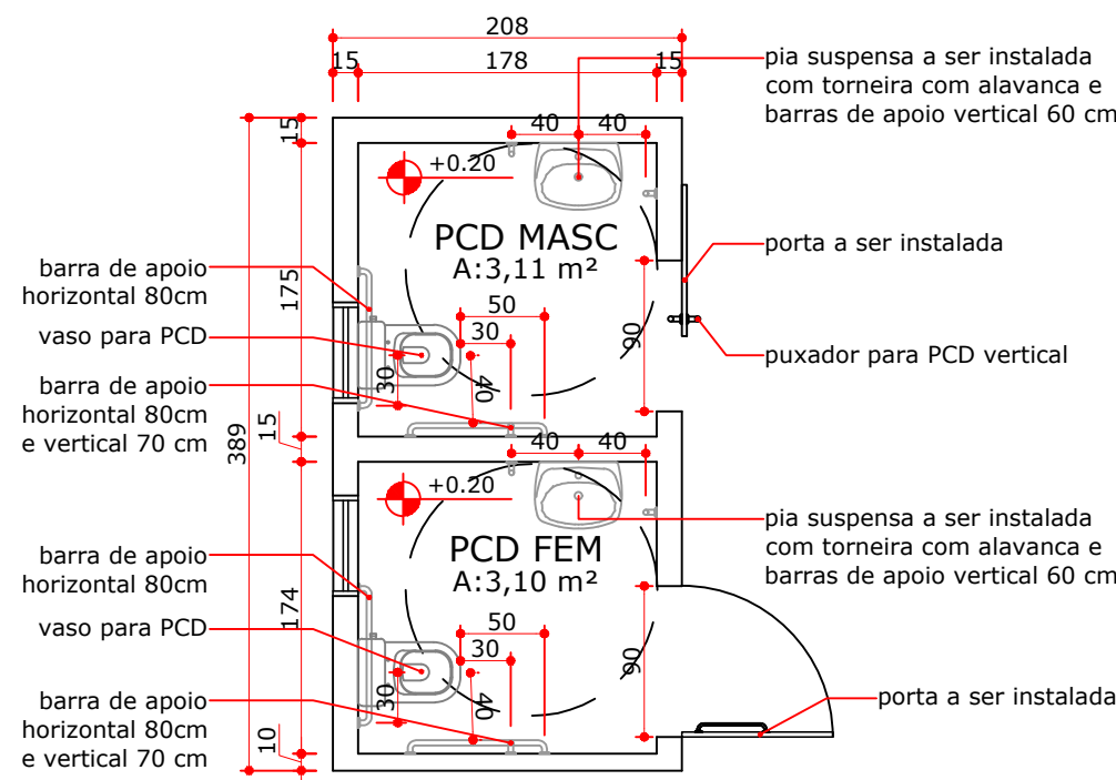
PLANTA MODIFICAÇÕES ESCALA 1:50
