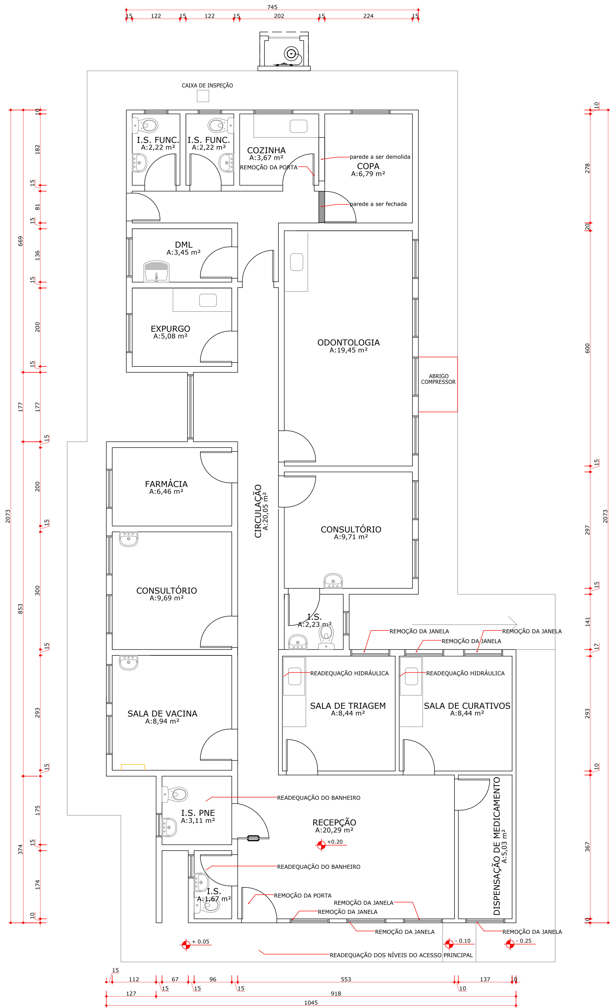
PLANTA INDICAÇÕES DE READEQUAÇÕES ESCALA 1:50
